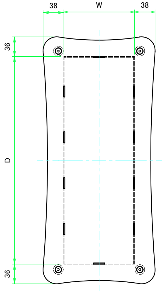
上カバー / Top cover
